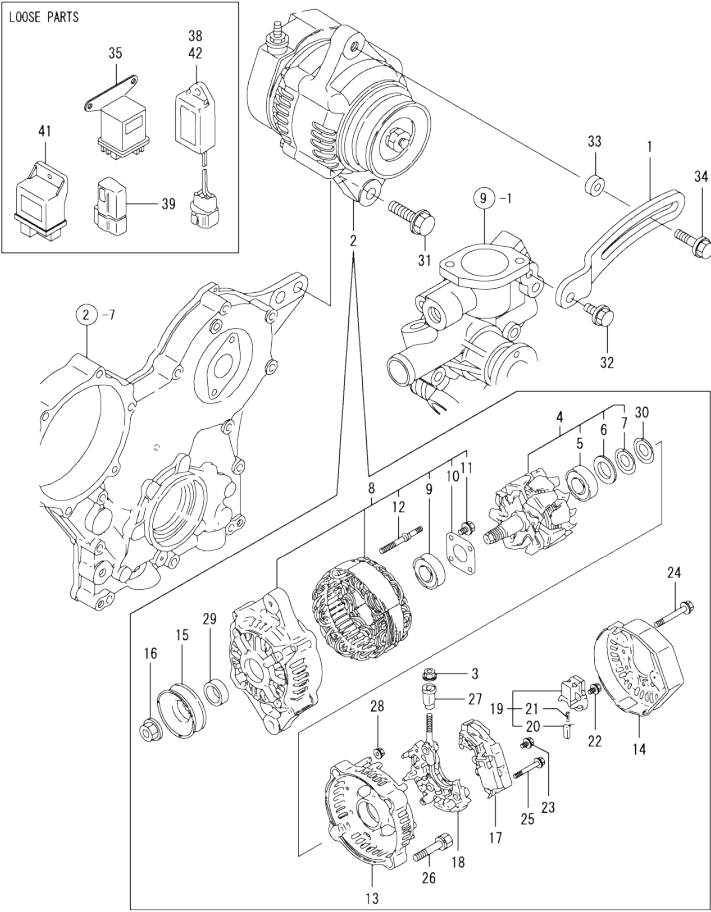
Fig.15. GENERATOR
